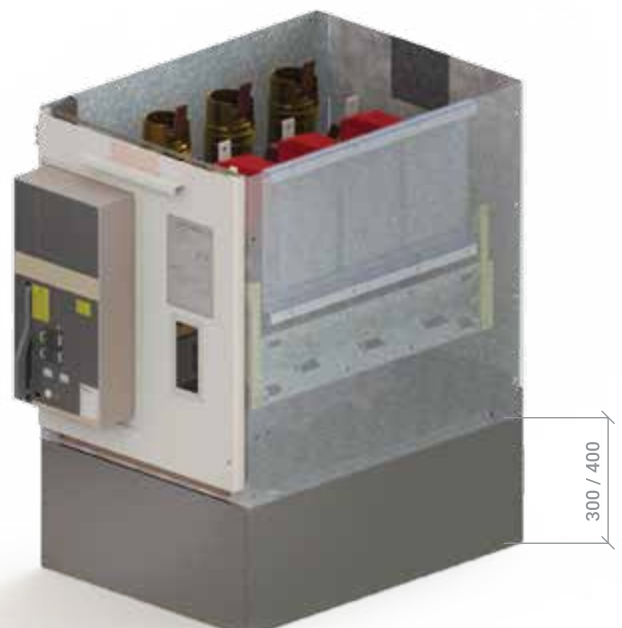
Zócalo para alineación de celdas y para usar como conducto de cables
